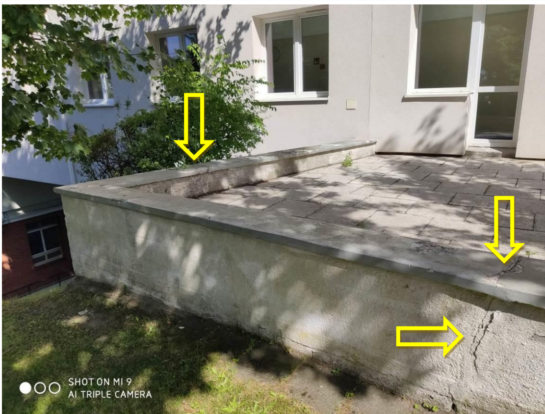
Zdjęcie nr 16 – Pęknięcia murku oporowego przy tarasie obok segmentu B od strony płd.
