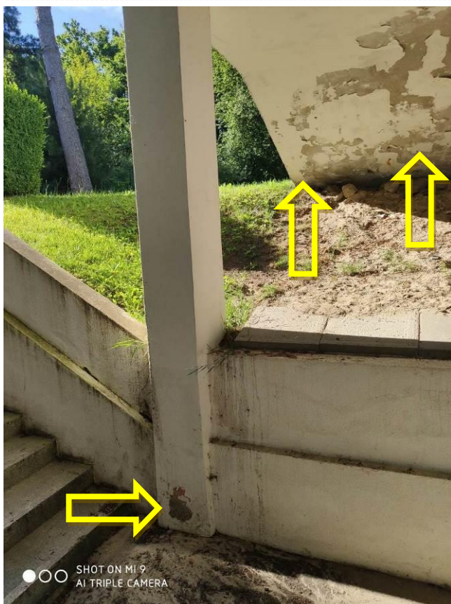
Zdjęcie nr 08 – Pęknięcia i odspojenia tynków na schodach głównych do segmentu C
